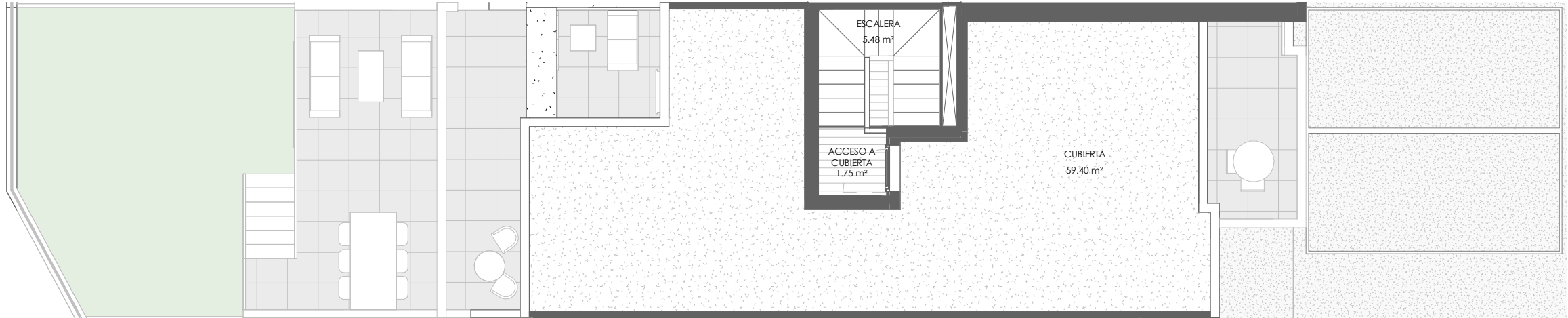
PLANTA CUBIERTA
