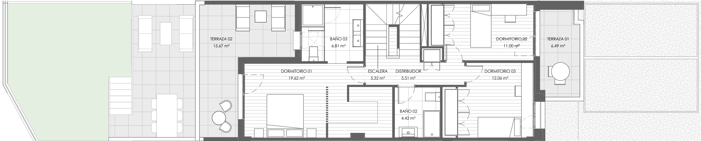
PLANTA PRIMERA
